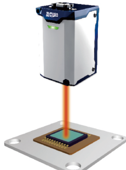
撮像素子の傾き測定
