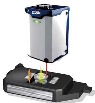
レンズの傾き測定
