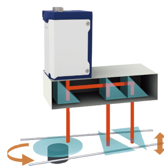
モータとシャフトの平行測定
